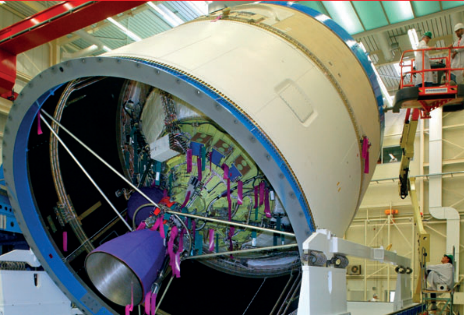
Antriebsaggregat EADS
