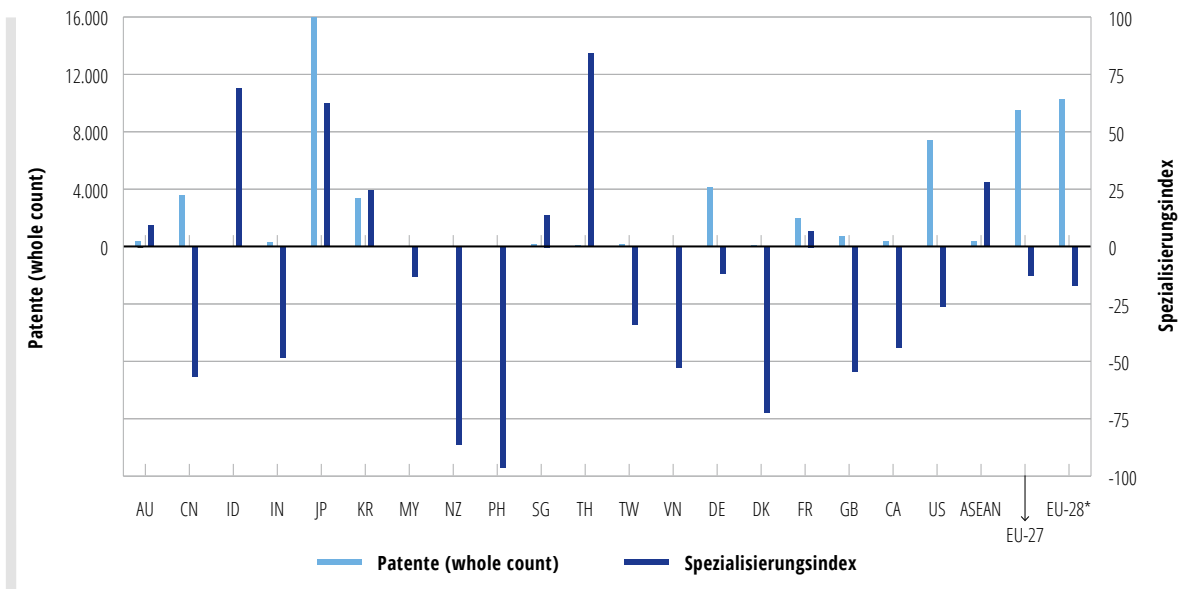
ABBILDUNG A18: Patentanmeldungen KETS - neuartige Werkstoffe, Summe 2015-17
